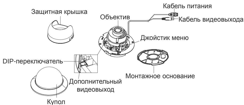
Рис. 1.1. Внешний вид видеокамеры
