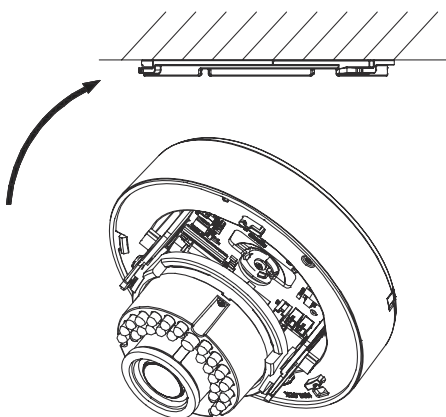
Рис. 2.3. Крепление видеокамеры к потолку
