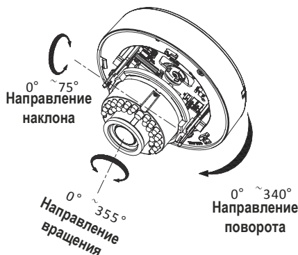
Рис. 2.4. Регулировка угла обзора
