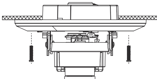
Рис. 2.6. Установка видеокамеры на креплении
