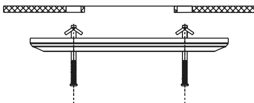
Рис. 2.5. Установка крепления в потолок
