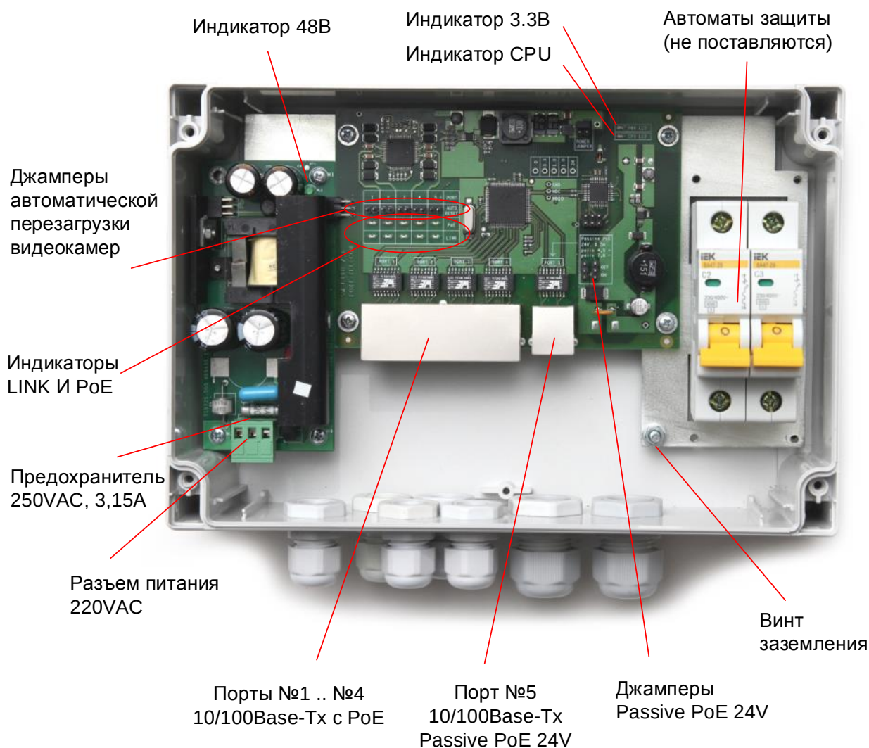
Рис. 2.2. Расположение элементов PSW -LITE
