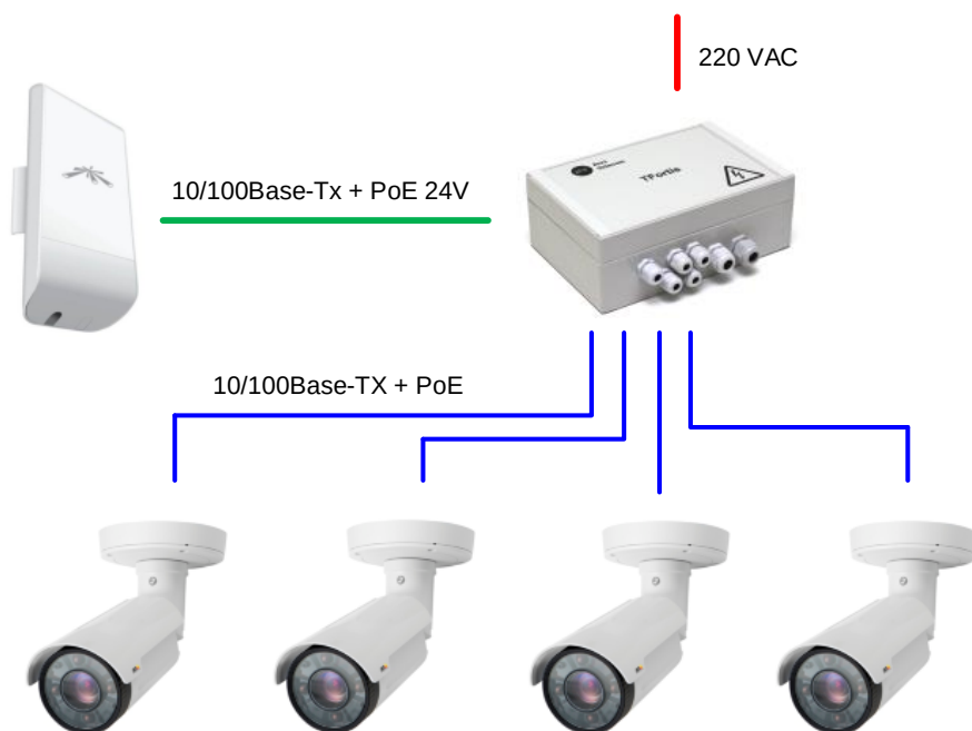
Рис. 1-2. Схема подключения PSW-LITE по Wi-Fi
