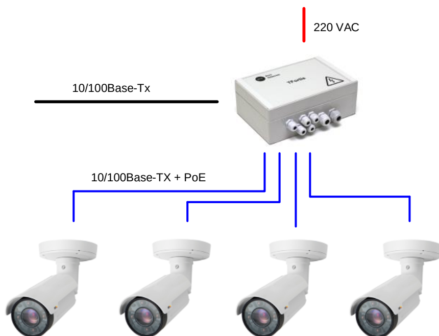
Рис. 1-1. Схема подключения PSW-LITE по витой паре
