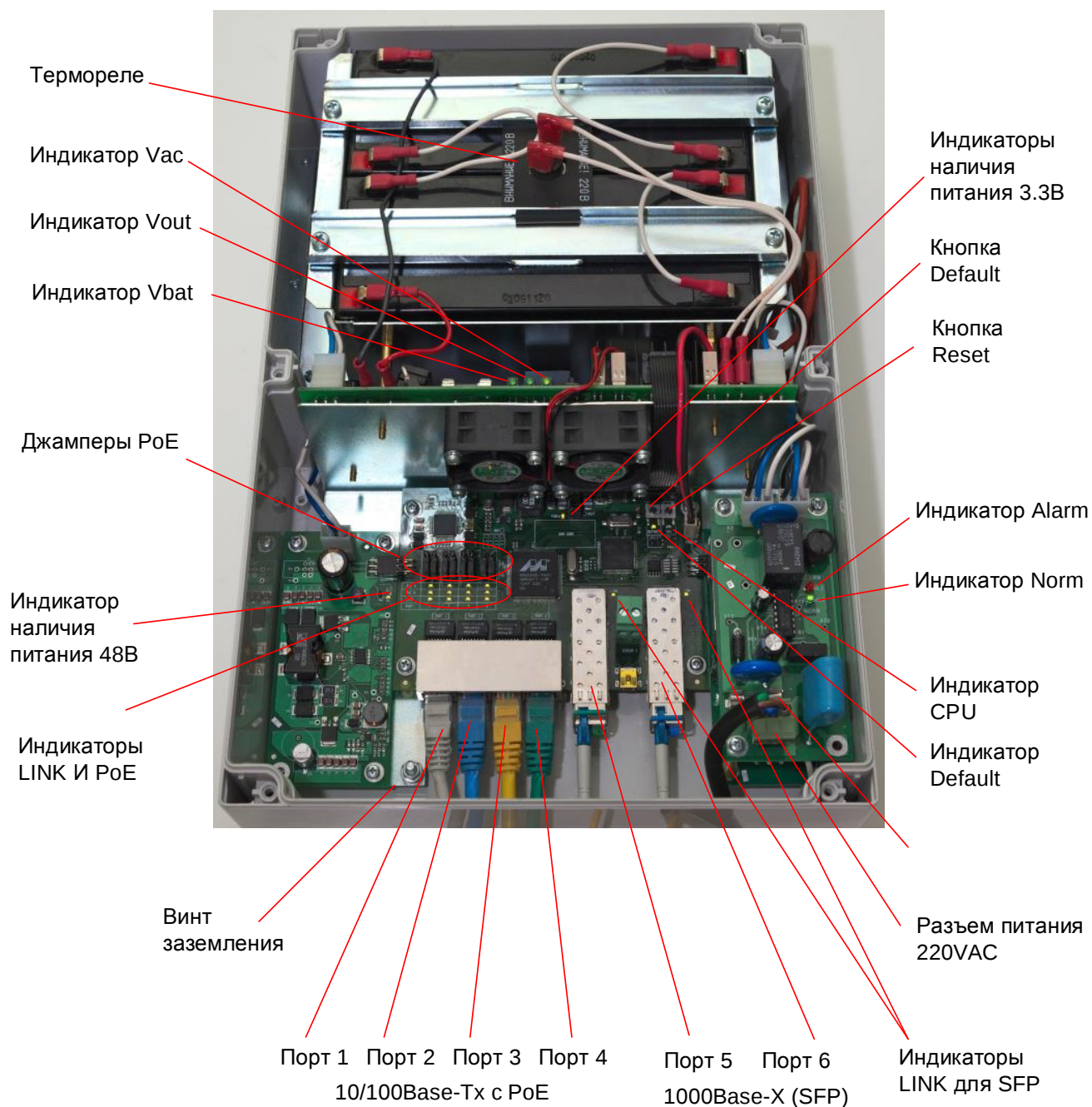
Рис. 2.2-2. Расположение элементов PSW -2G4F-UPS
