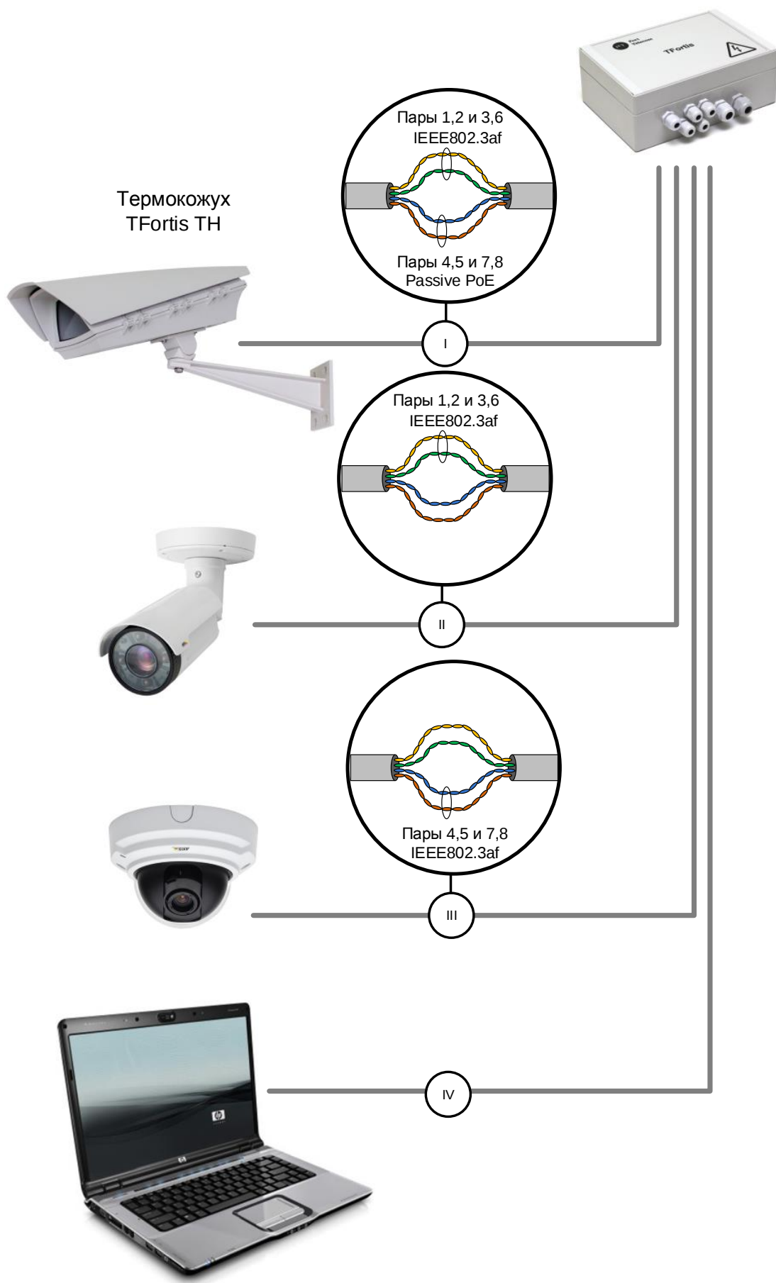
Рис. 2.3. Схема питания по PoE для разных случаев
